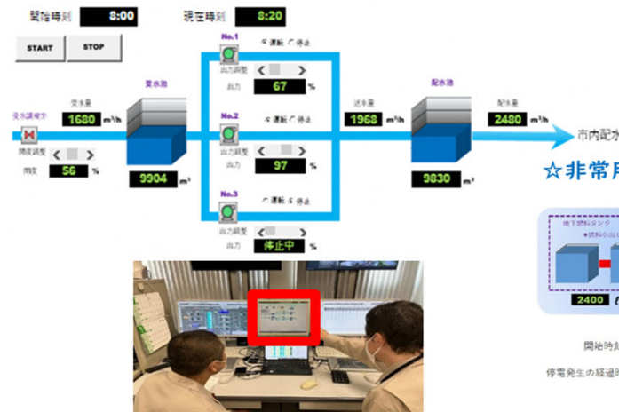
☆運転管理委託業者の水運用シミュレータを活用した教育風景
