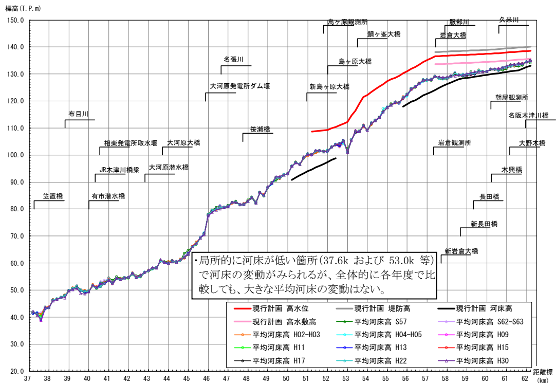
図 1.3.3 木津川平均河床高縦断面図
