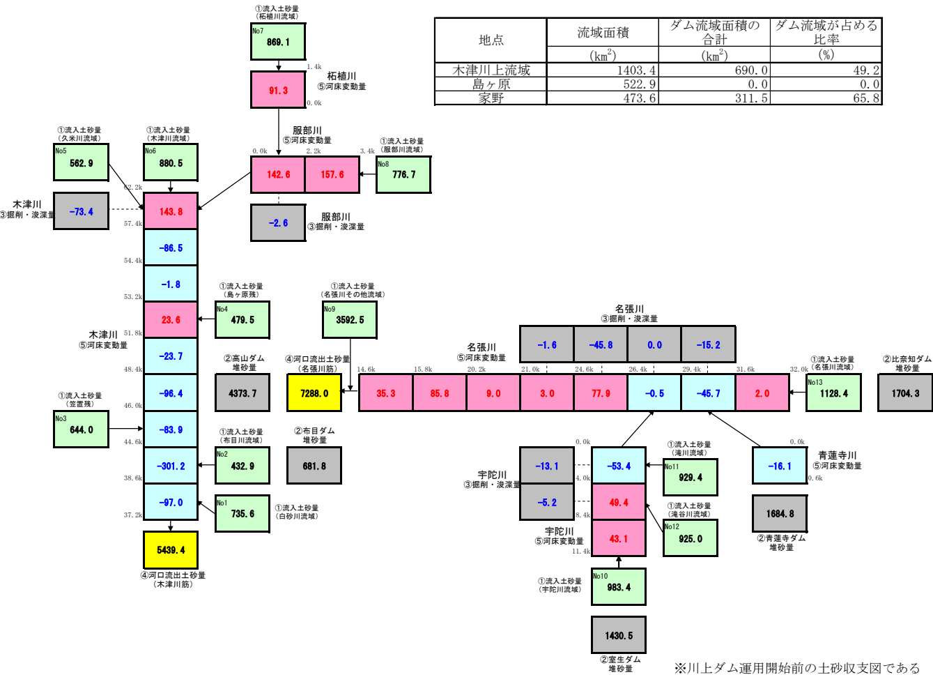
図 1.4.1 木津川上流域における土砂収支図（土砂動態マップ）
