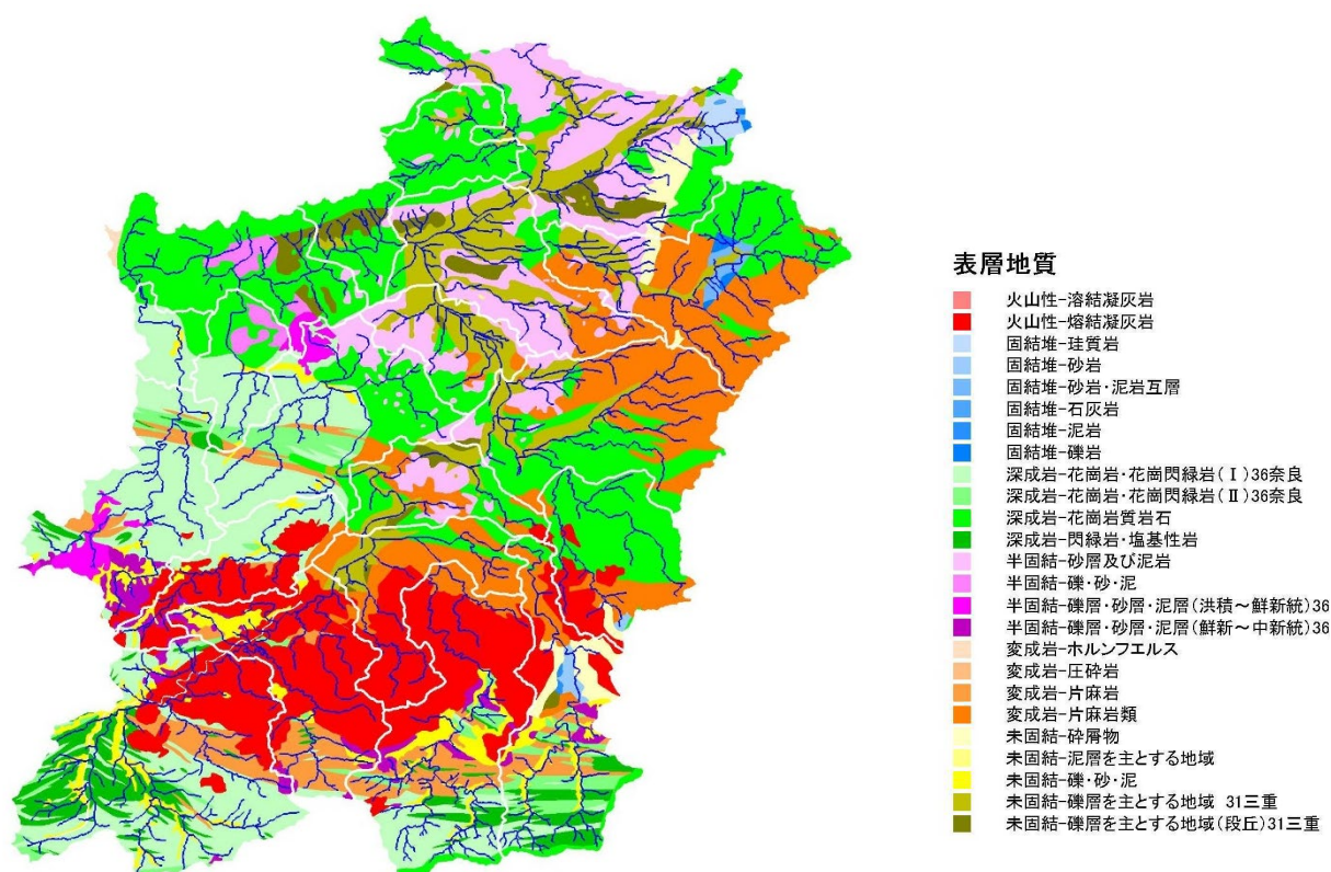
図 1.3.2 木津川上流域表層地質図（出典：土地分類基本調査）
