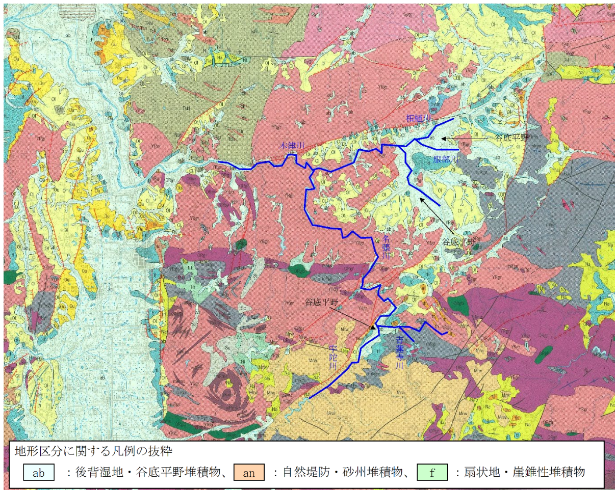
図 1.3.1 地形・地質区分図
