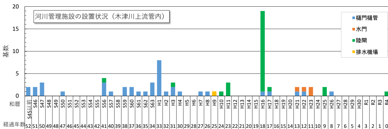
図 2.3.1 木津川上流における河川管理施設の設置状況
