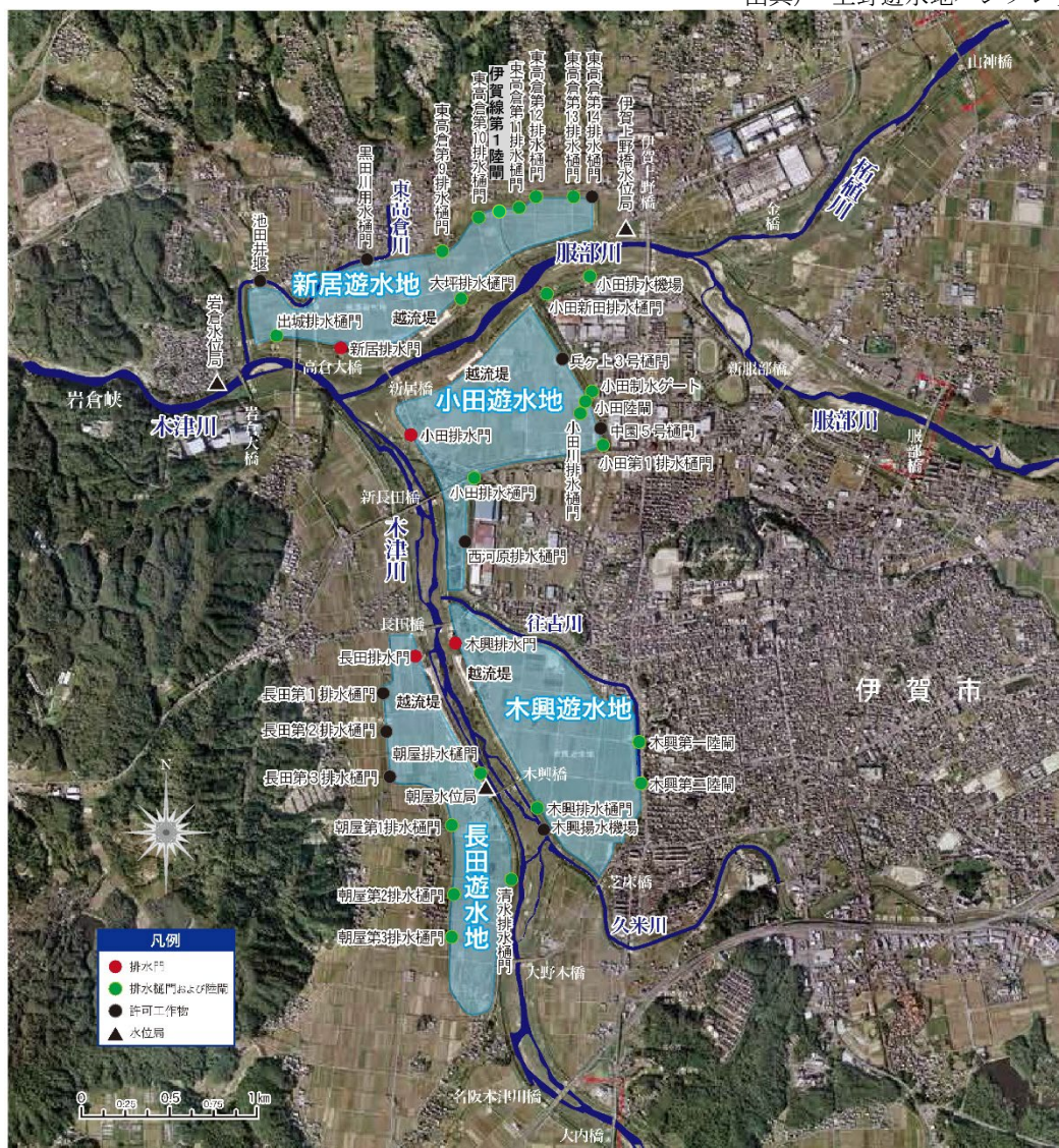
図 2.1.1 上野遊水地全景
