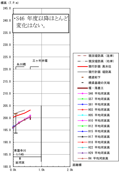
図 1.3.8 青蓮寺川平均河床高縦断図
