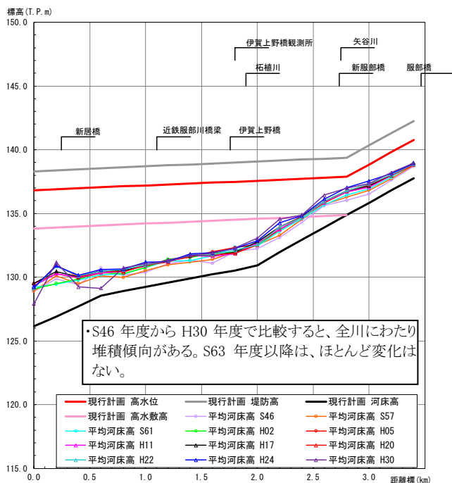
図 1.3.4 服部川平均河床高縦断面図
