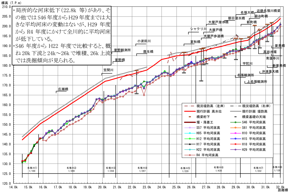
図 1.3.6 名張川平均河床高縦断図
