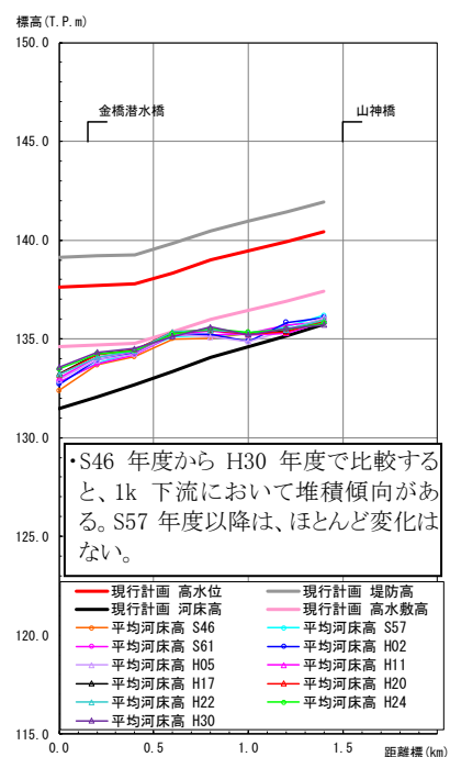
図 1.3.5 柘植川平均河床高縦断面図
