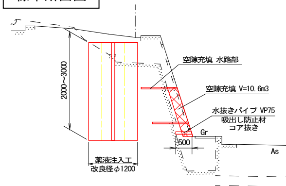
標準断面図
