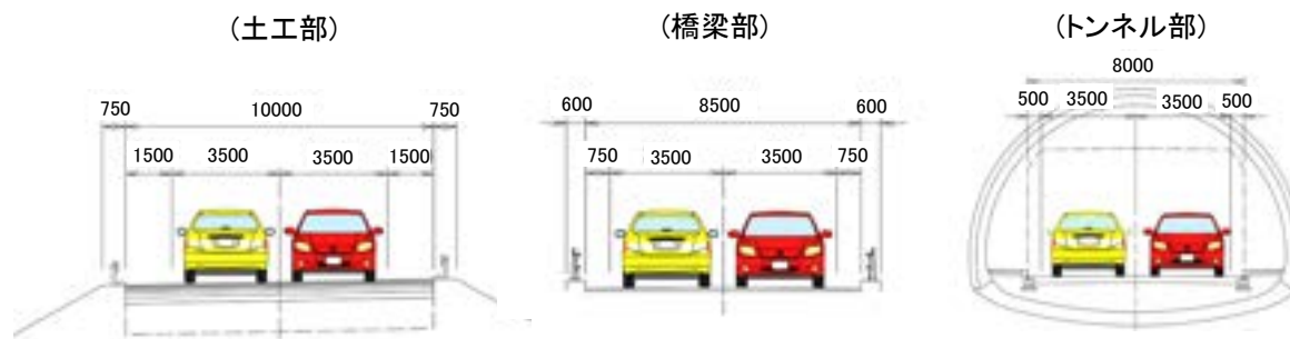
標準断面図
