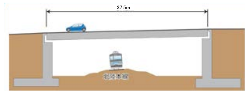
計画側面図
