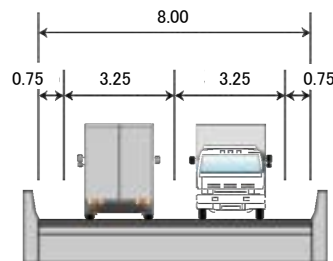
計画断面図
