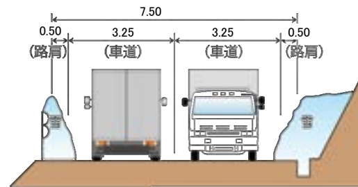
現況断面図
