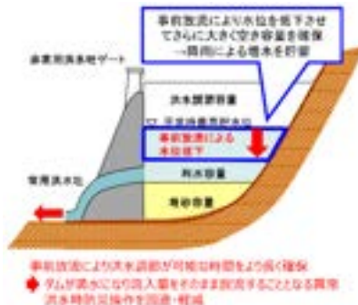
多目的ダムにおける事前放流
